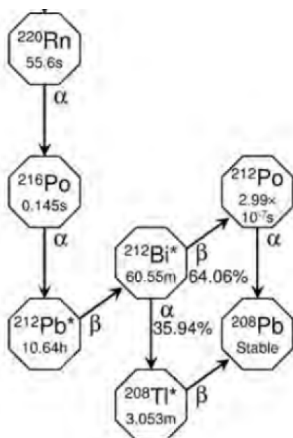
Figur 1: Desintegrasjon av radon-220 til bly-208, inkludert halveringstider.
