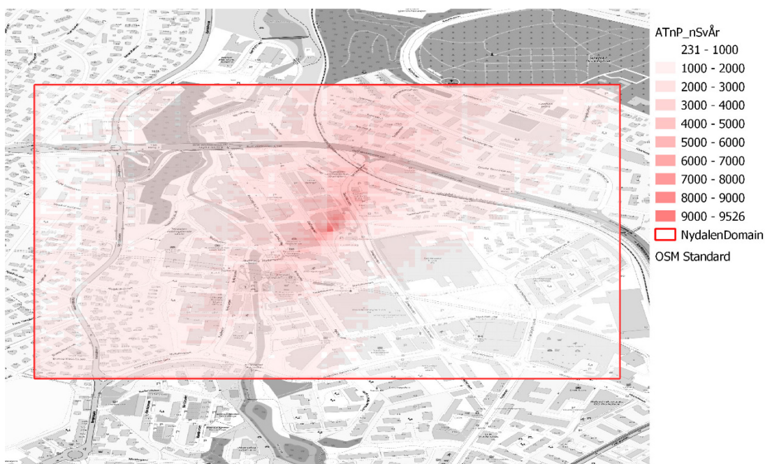
Figur 12: Beregnet eksponeringsdose fra thorondøtre ( A_{TnP} ) antatt kontinuerlig opphold i området. Enhet: nSv/år.
