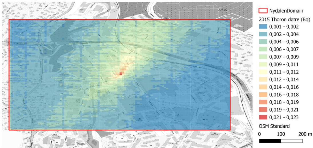
Figur 7: Modellert aktivitetskonsentrasjon av thorondøtre for laget nærmest bakken for 2015 (i Bq\ m^{-3} ). Tallene er gjennomsnittskonsentrasjoner av thorondøtre for nærområdet som dekker Nydalen.
