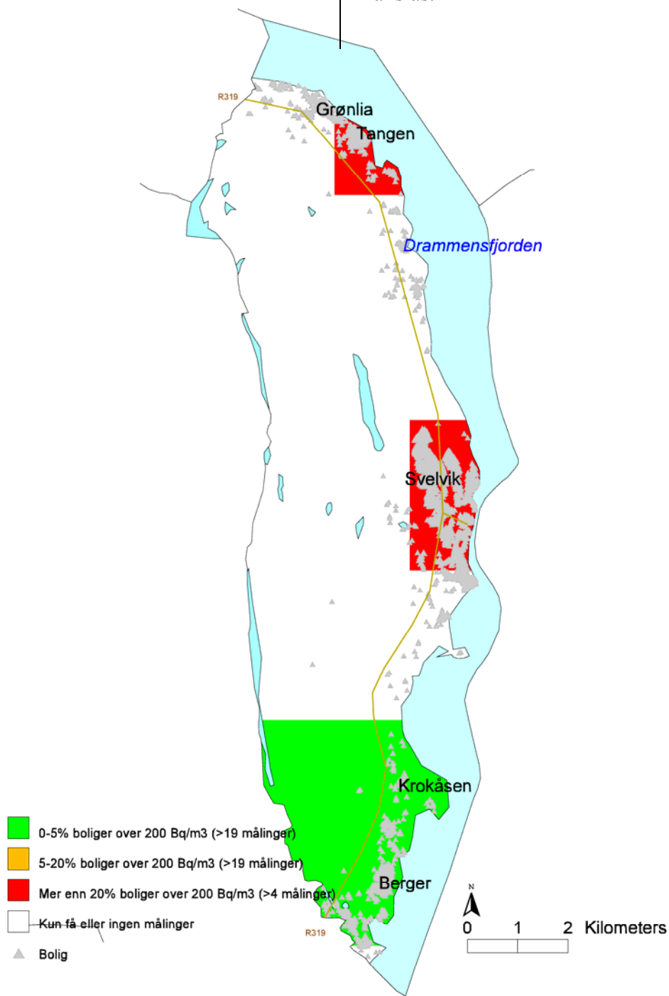
Figur 1: Områdekart for Svelvik kommune, basert på målinger i forbindelse med prosjektet RaMAP. Kartet er utarbeidet på grunnlag av 168 målinger.
