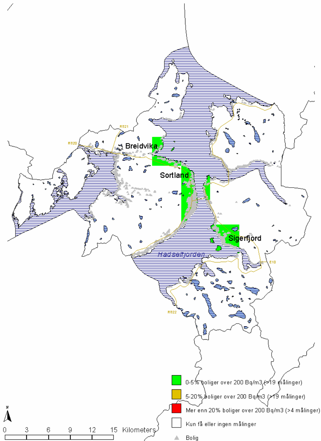
Figur 1: Områdekart for Sortland kommune. Oversikt over måleresultater fra "Radon 2000/2001", der radonkonsentrasjonen i inneluft ble målt i 8 % av boligmassen i kommunen.
