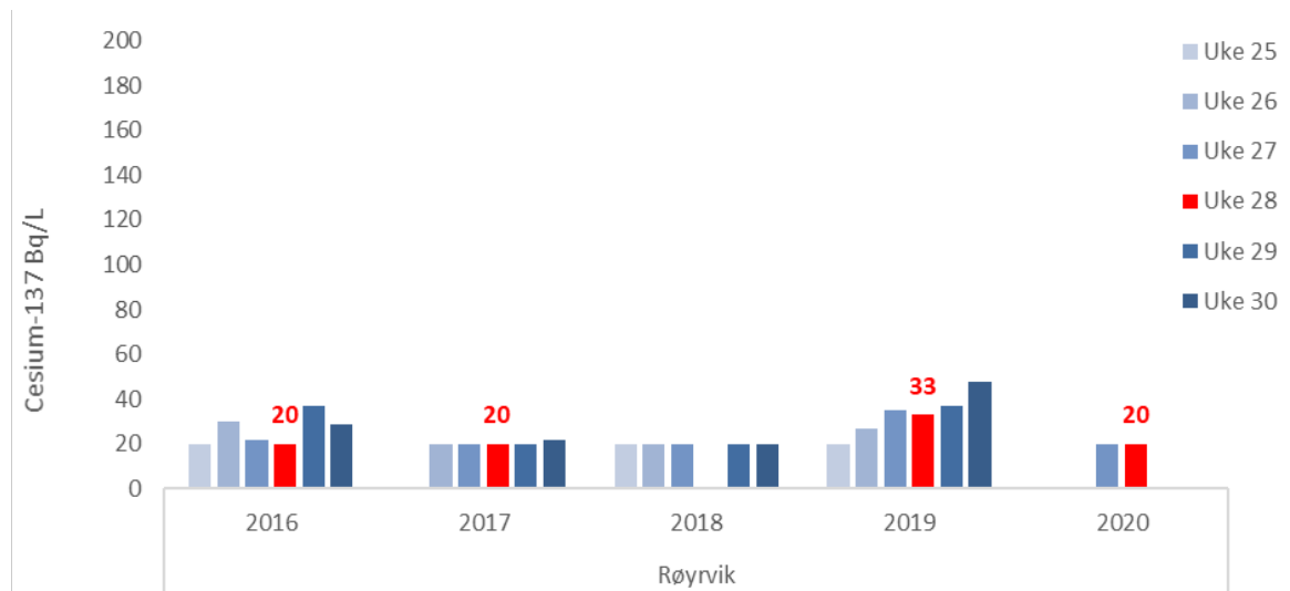
Figur 3: Konsentrasjon av cesium-137 (Bq/l) i geitemelk fra besetning 5043 0065 (tidl. 1739 3113) i Røyrvik.
