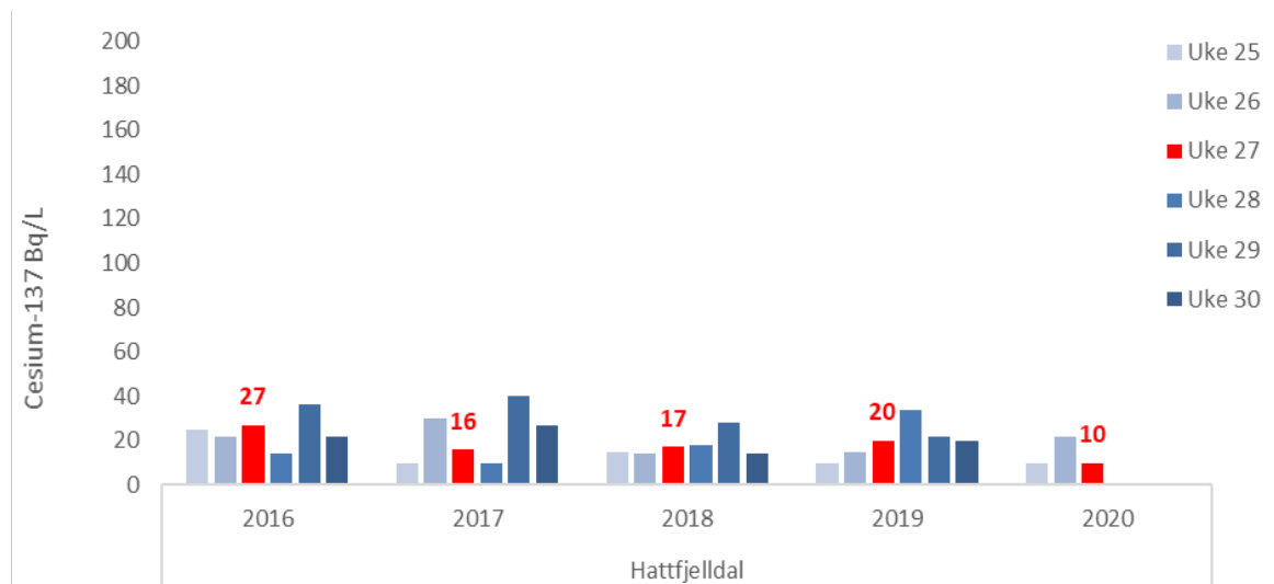
Figur 4: Konsentrasjon av cesium-137 (Bq/l) i kumelk fra besetning 1826 0217 i Hattfjelldal. Denne er i 2020 erstattet med besetning 1826 0189 som beiter i samme område.
