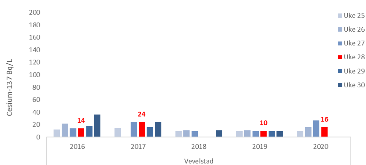
Figur 5: Konsentrasjon av cesium-137 (Bq/l) i kumelk fra besetning 1816 0125 i Vevelstad.
